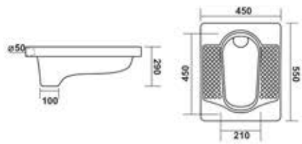
5005-AQUA PAN 21" L 550 W 450 H 290mm
